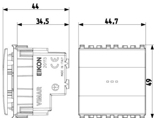
Vista ingombri
