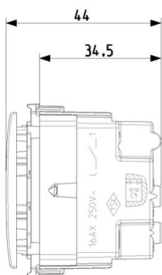
Vista ingombri
