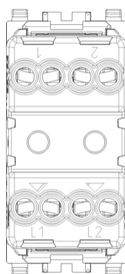
Vista posteriore
