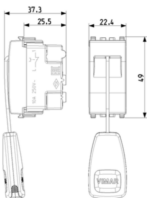
Vista ingombri
