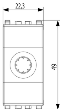
Vista ingombri
