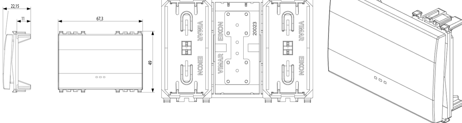
Vista ingombri
