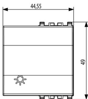
Vista ingombri
