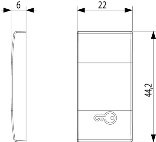
Vista ingombri
