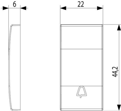
Vista ingombri
