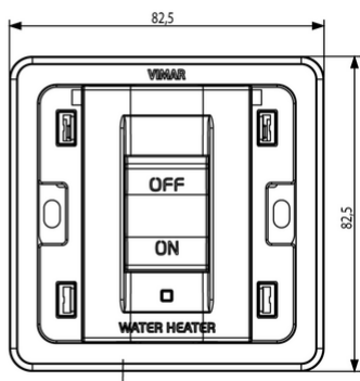
Vista ingombri
