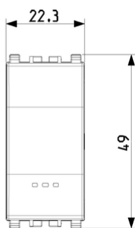
Vista ingombri
