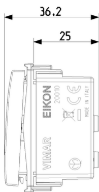
Vista ingombri
