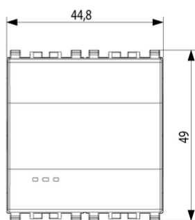
Vista ingombri
