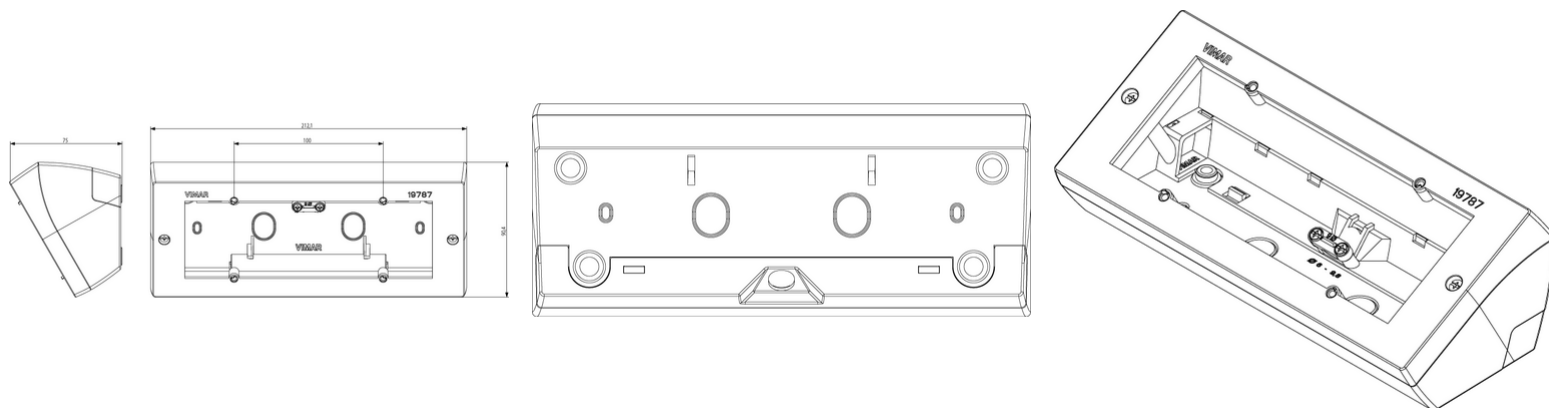
Vista ingombri
