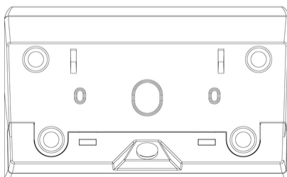
Vista posteriore
