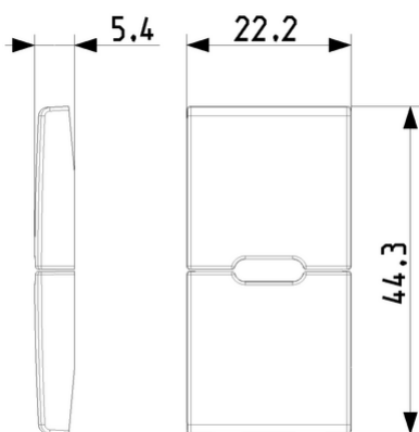
Vista ingombri
