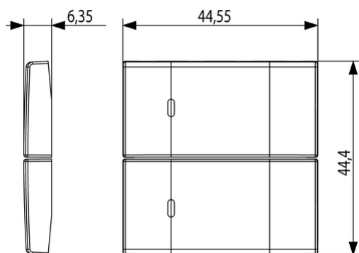
Vista ingombri
