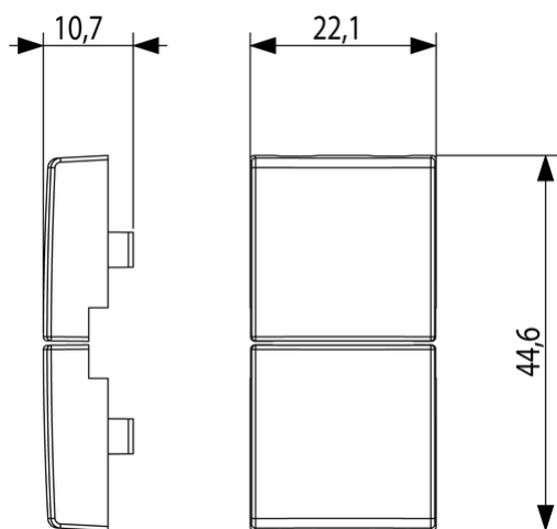
Vista ingombri
