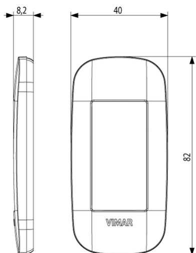
Vista ingombri
