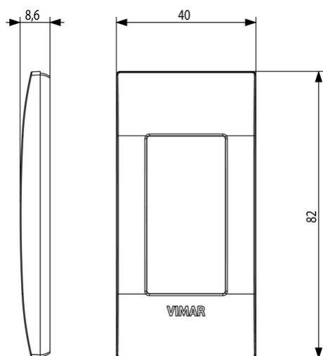
Vista ingombri
