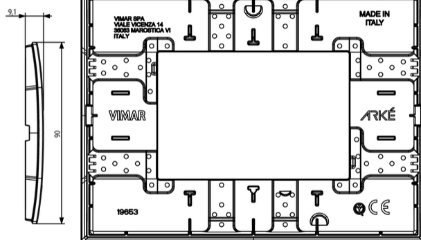
Vista posteriore
