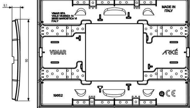
Vista posteriore
