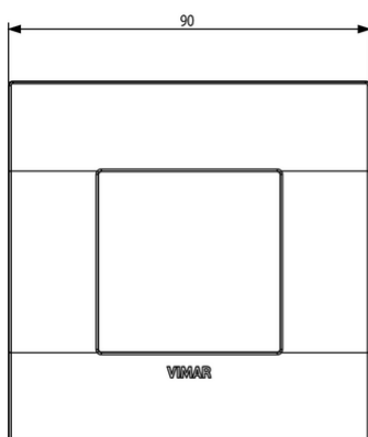
Vista ingombri
