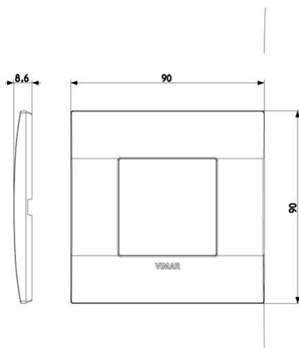
Vista ingombri
