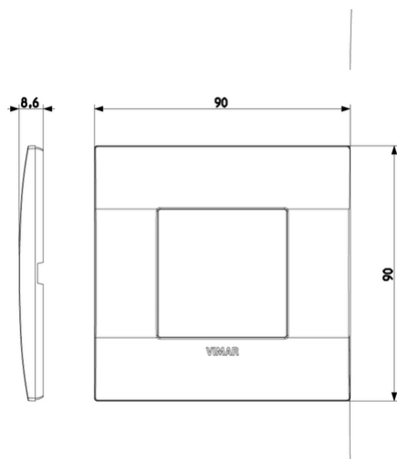
Vista ingombri
