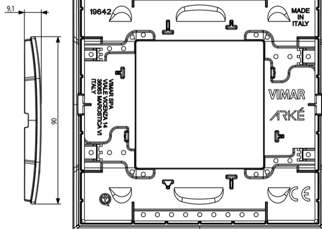
Vista posteriore
