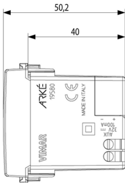
Vista ingombri
