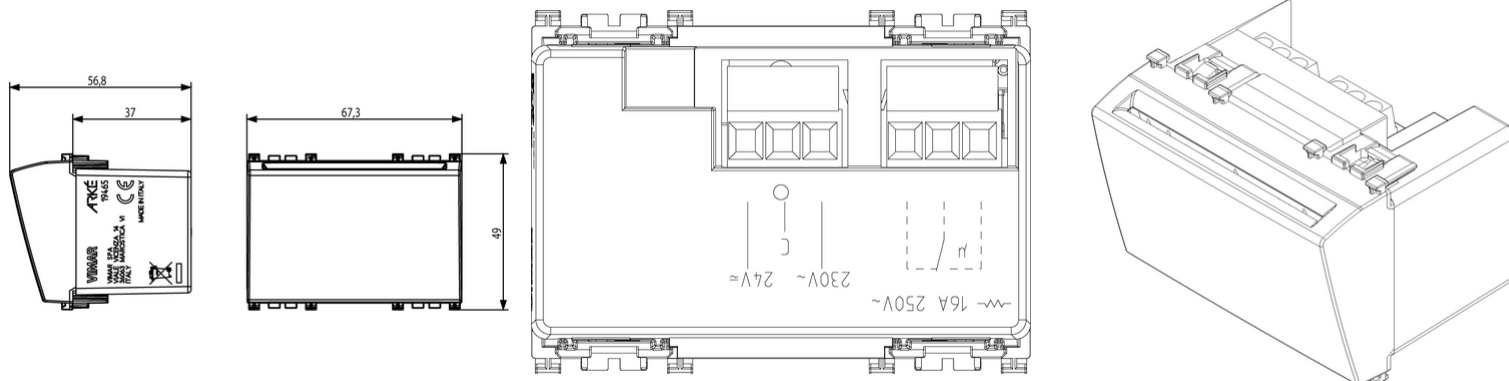
Vista ingombri
