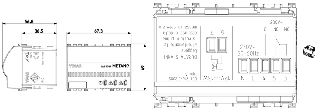
Vista ingombri
