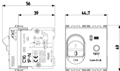
Vista ingombri
