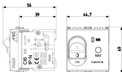
Vista ingombri
