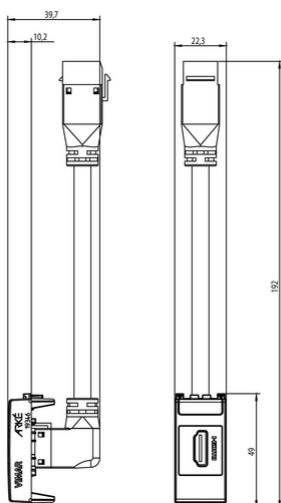
Vista ingombri
