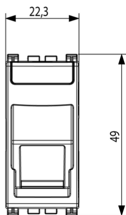
Vista ingombri
