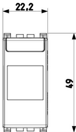
Vista ingombri
