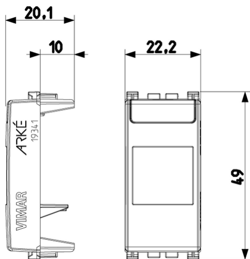
Vista ingombri
