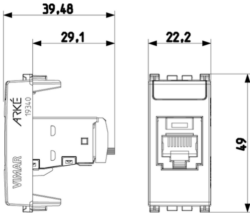
Vista ingombri
