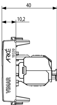
Vista ingombri
