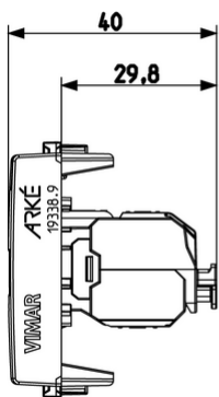
Vista ingombri
