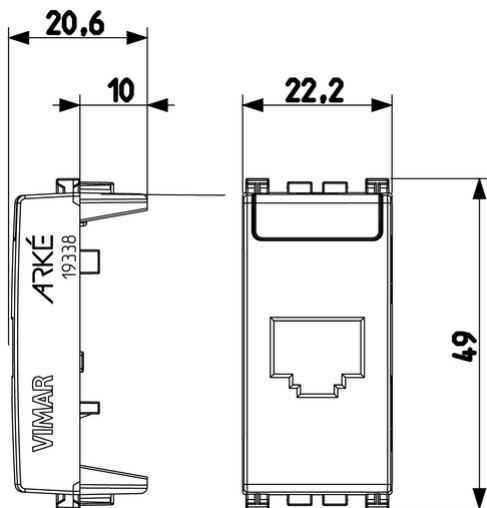
Vista ingombri
