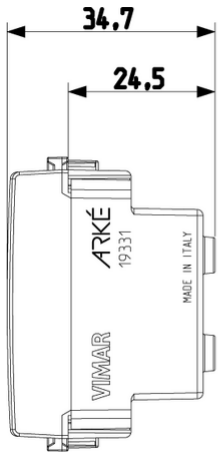
Vista ingombri
