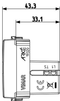
Vista ingombri
