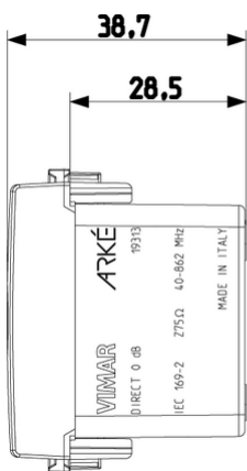
Vista ingombri
