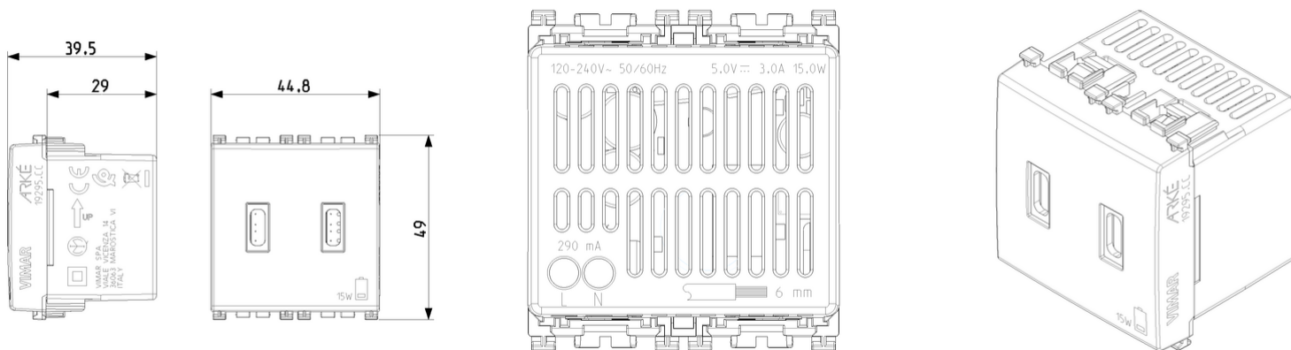
Vista ingombri
