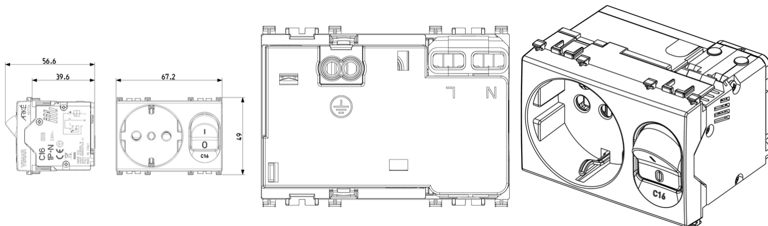
Vista ingombri
