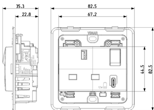
Vista ingombri
