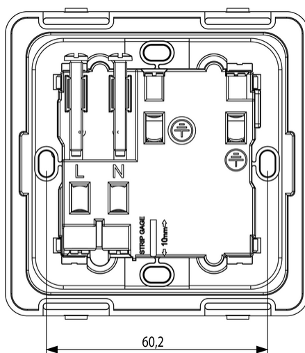
Vista posteriore
