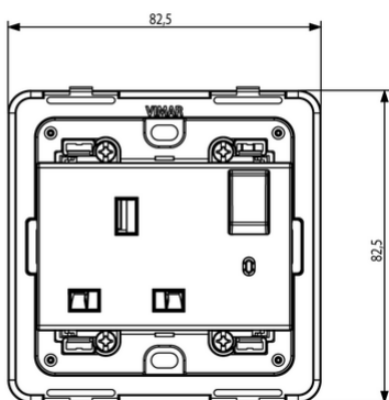
Vista ingombri
