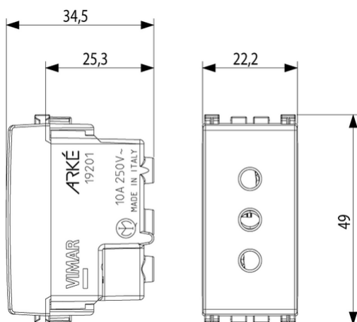
Vista ingombri
