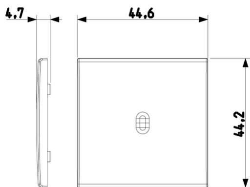
Vista ingombri
