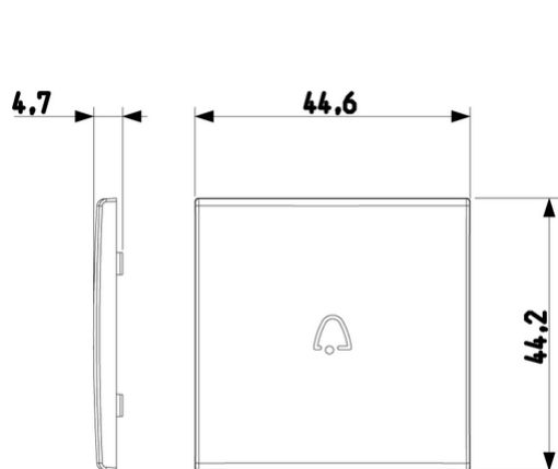
Vista ingombri
