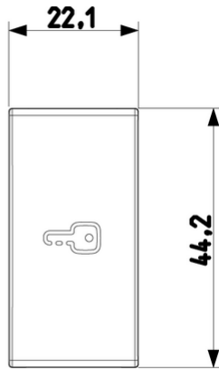
Vista ingombri
