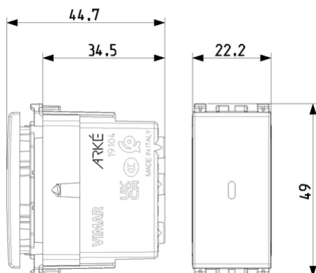
Vista ingombri
